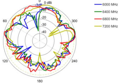
Elevation 2: 6000 – 7200 MHz
