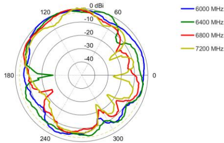
Elevation 2: 6000 – 7200 MHz
