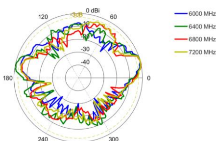
Elevation 2: 6000 – 7200 MHz
